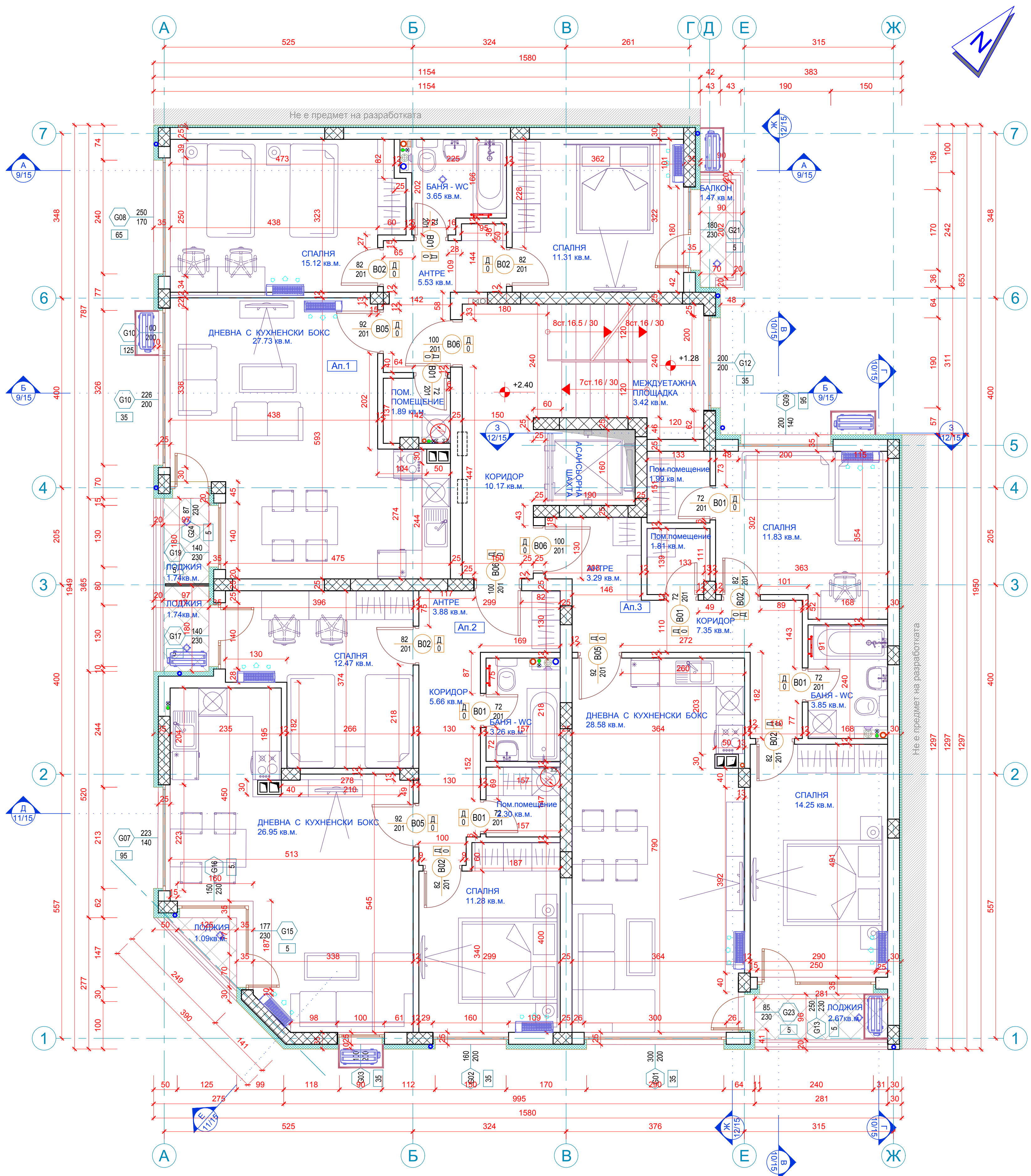
План на K+2.40 M1:50
