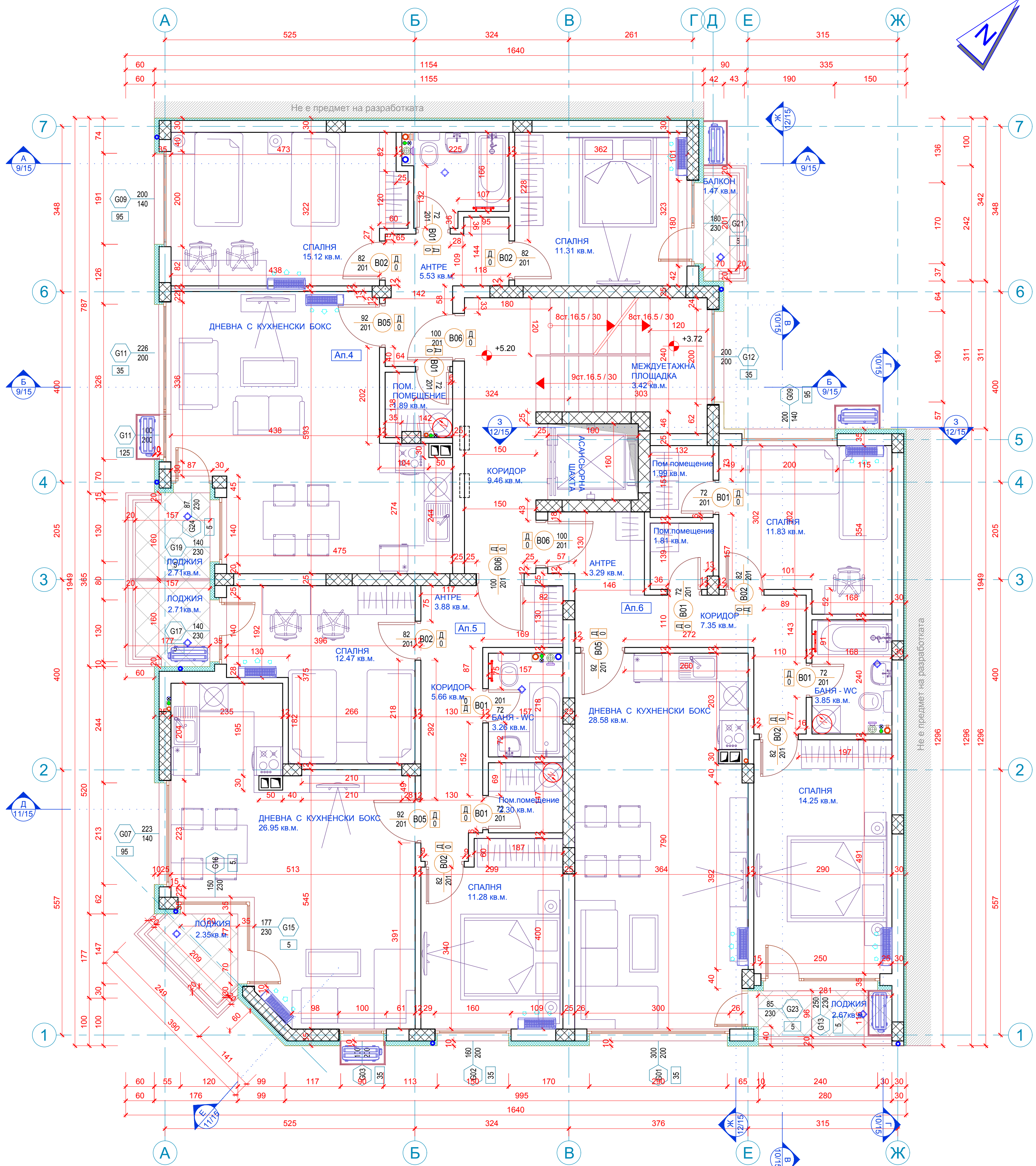
План на K+5.20 М1:50
