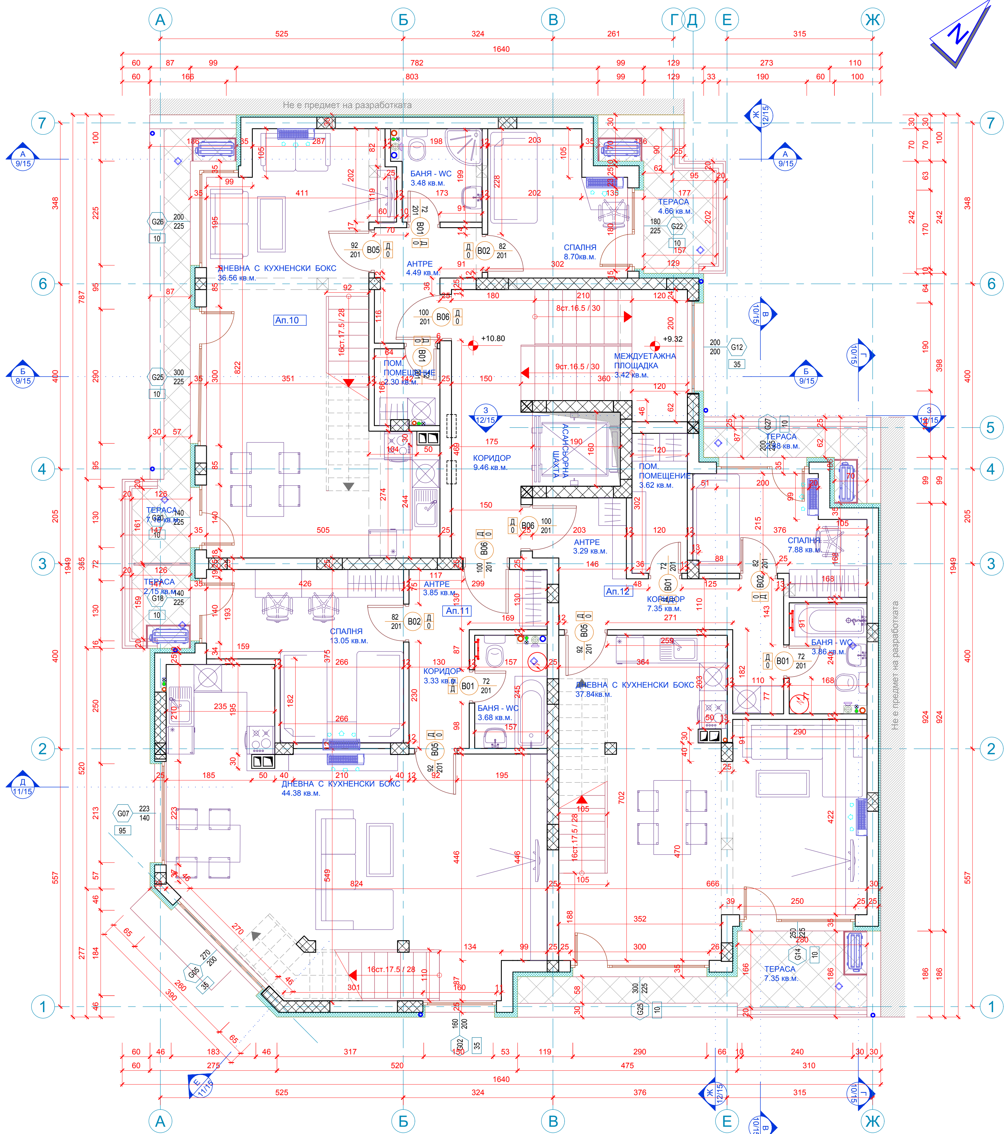
План на K+10.80 M1:50
