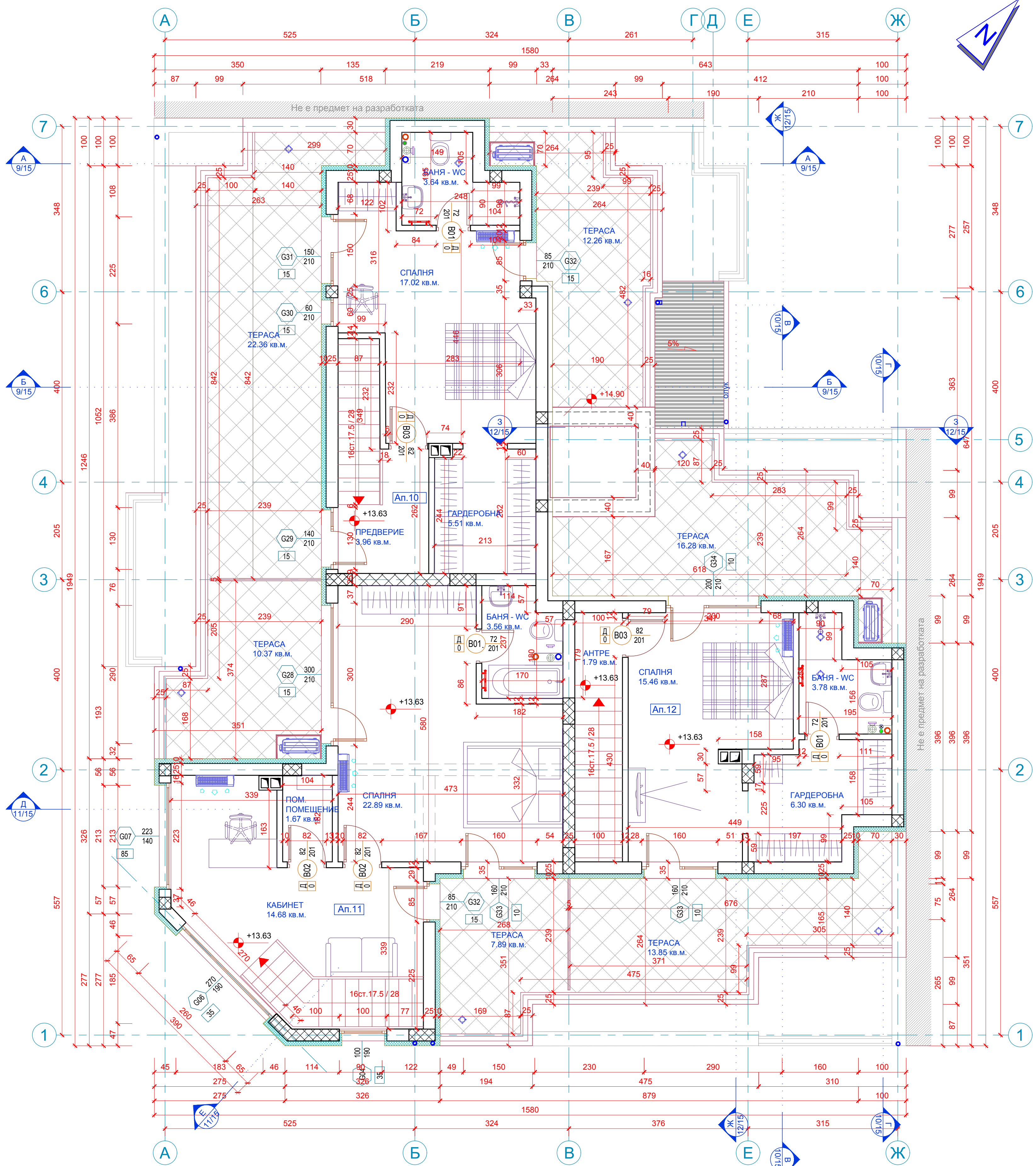
План на К+13.63 М1:50
