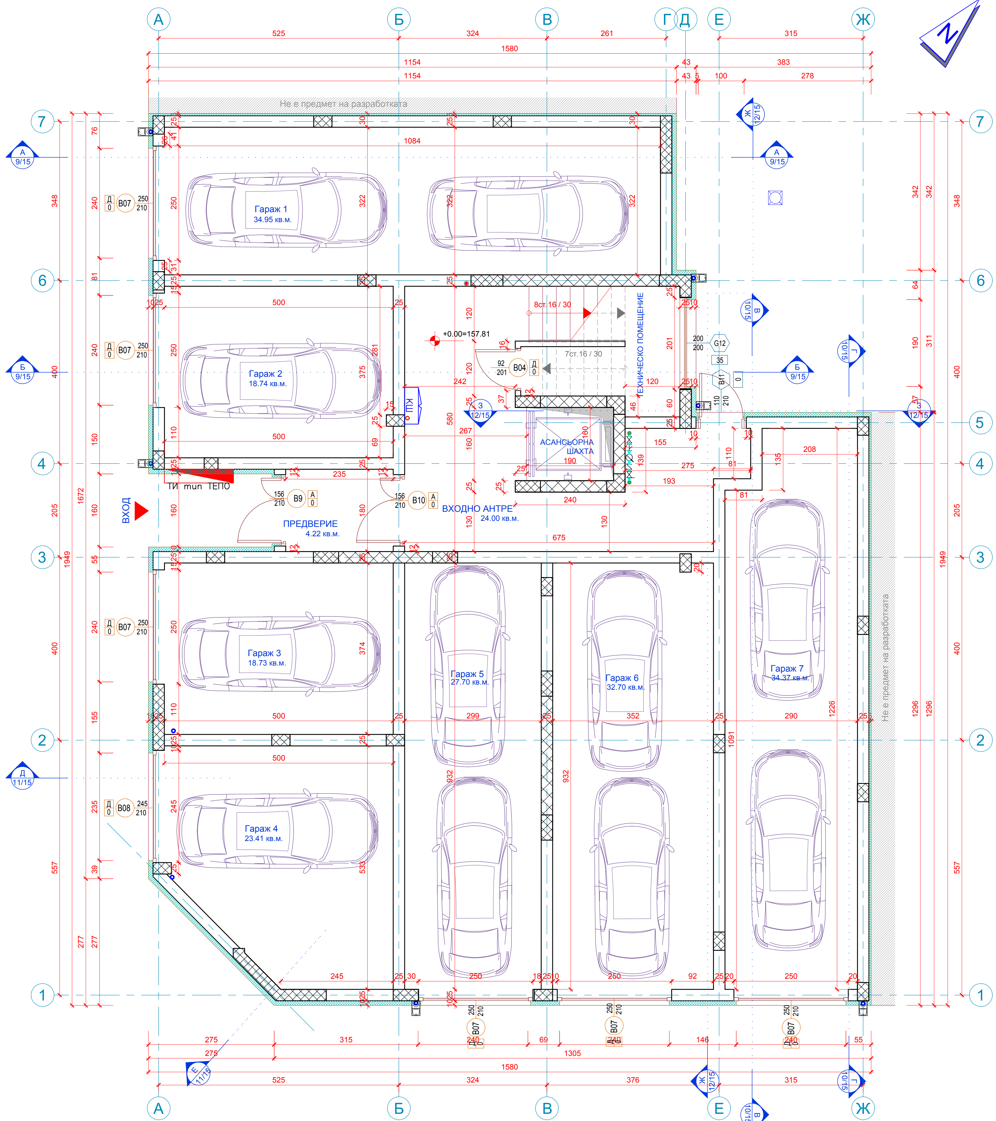
План на партер К+0.00 М1:50
